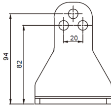
Beugel 1. (montage op paal)
